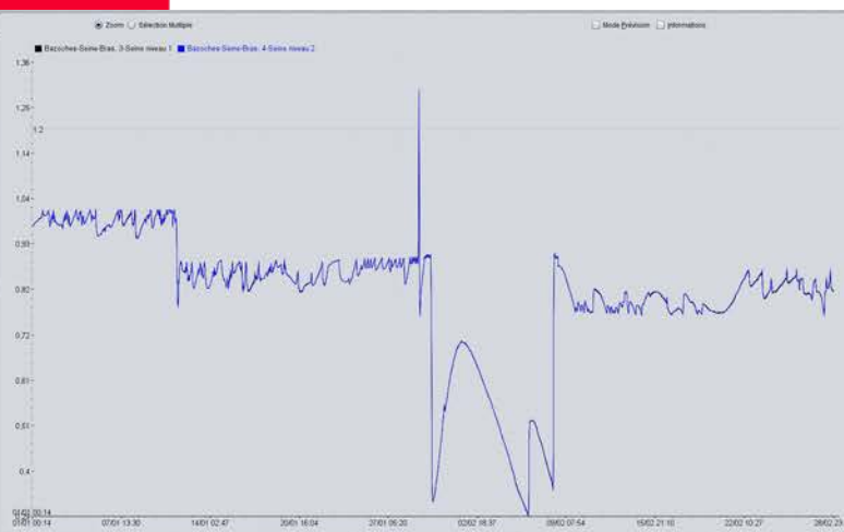
Bazoches-les-Bray, crue 2018 – le barrage de la grande bosse est abattu au moment du pic de crue
