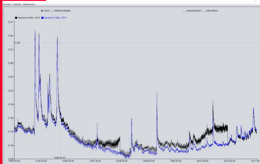
Nesles-la-vallée – été 2018- entartrage du bulle à bulle
