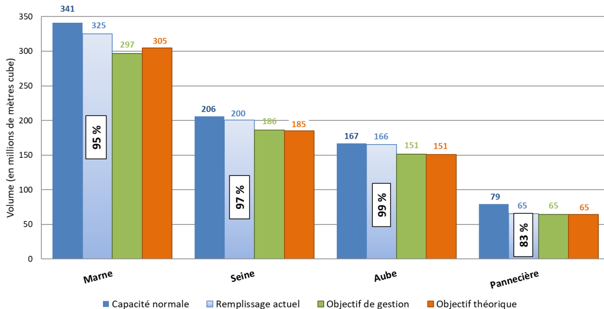
Remplissage des lacs-réservoirs au 15/07/2024
