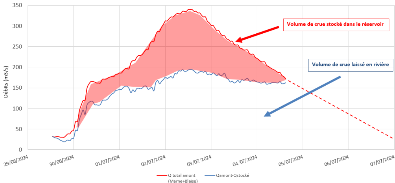
Réservoir Marne _ Gestion crue juillet 2024
